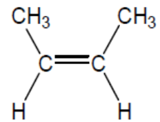
cis-2-Butene
